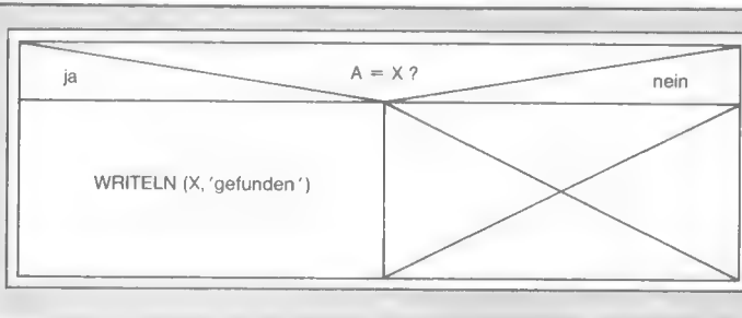
Bild 3. Struktogramm der einfachen IF-Anweisung
